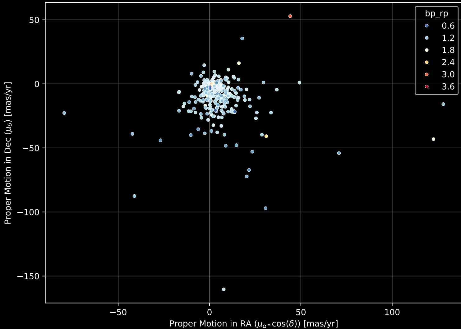
GALAH DR4 Field: [6777] Proper Motion Diagram (n= 510)
