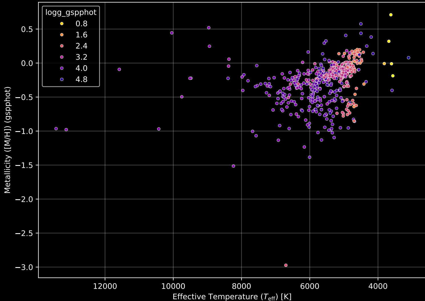
GALAH DR4 Field: [6777] Stellar Population Parameters (n= 510)
