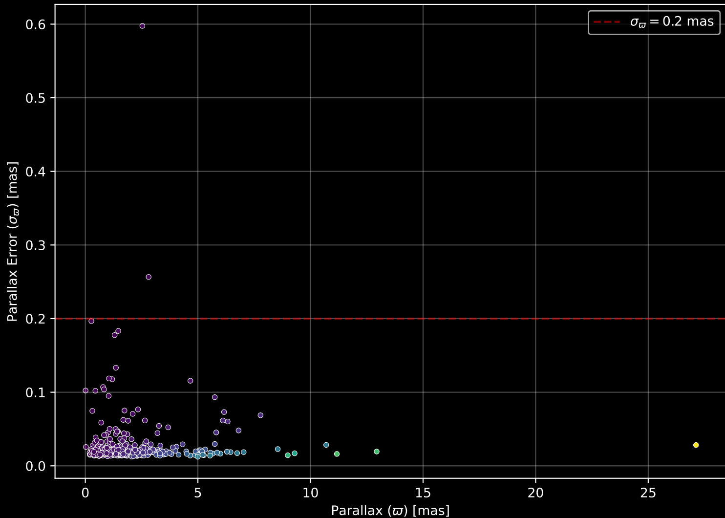
GALAH DR4 Field: [6777] Parallax Quality (n= 510)
