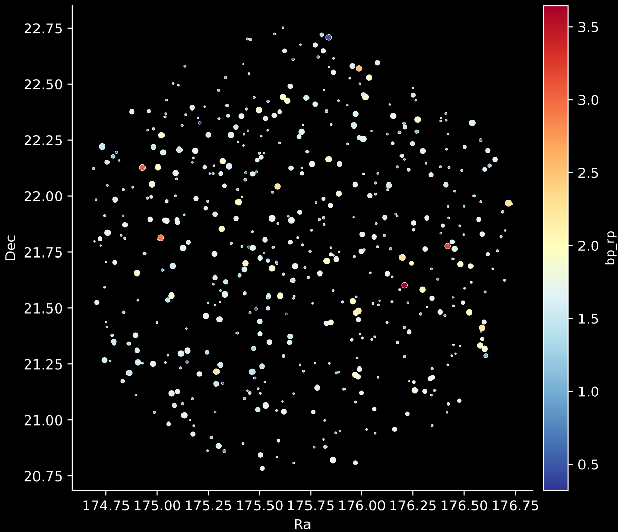
GALAH DR4 Field: [6777] Stars: 510
